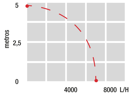
DIAGRAMA CAPACIDAD CAUDAL
